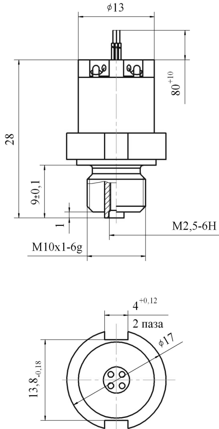
Рисунок Б.1 – Тензопреобразователи серии Н конструктивного исполнения 1
