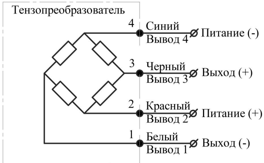
Рисунок А.1 – Схема «Замкнутый мост»
